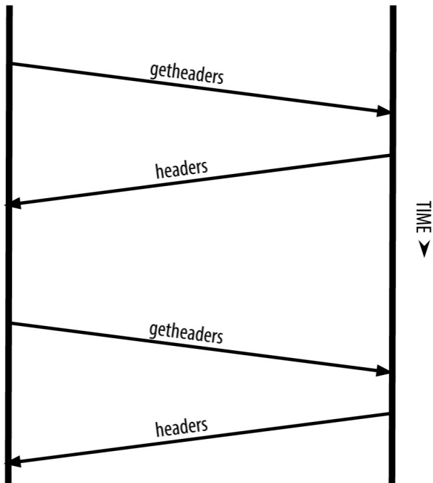
Figure 7. Nodo SPV sincronizando las cabeceras de bloque
