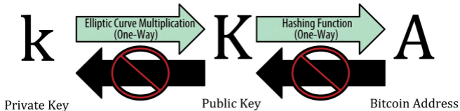
Figure 1. Clave privada, clave pública y dirección bitcoin
