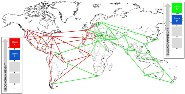
Figure 4. Visualización de un evento bifurcación en la cadena de bloques: se propagan dos bloques, seccionando la red
