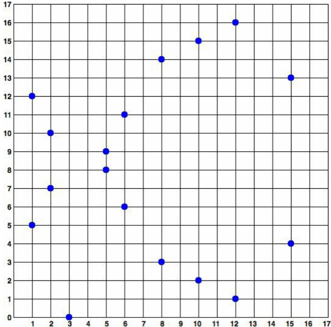
Figure 3. Criptografía de curva elíptica: visualizando una curva elíptica sobre F(p) , con p=17 Así que, por ejemplo, el siguiente es un
