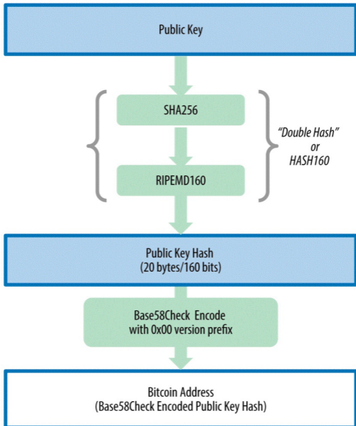
Figure 5. Clave pública a dirección bitcoin: conversión de una clave
