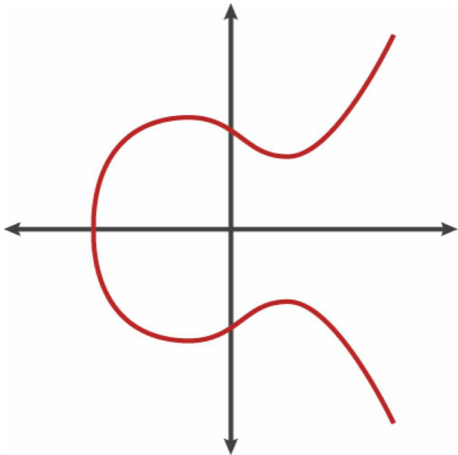
Figure 2. Una curva elíptica
