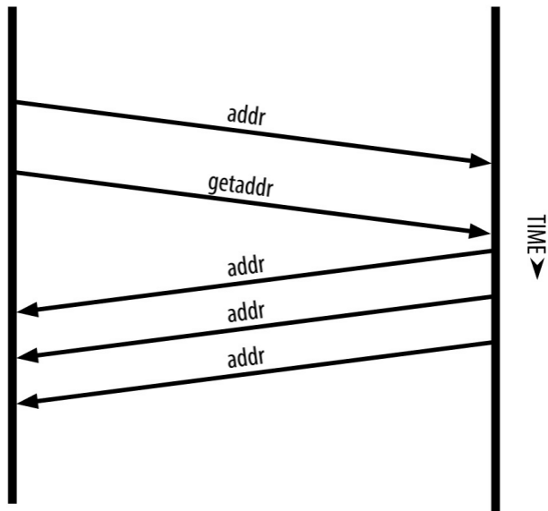
Figure 5. Descubrimiento y propagación de la dirección
